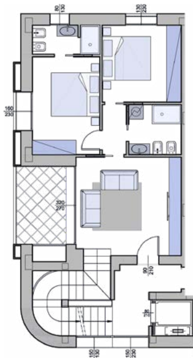
PIANO TERZO
